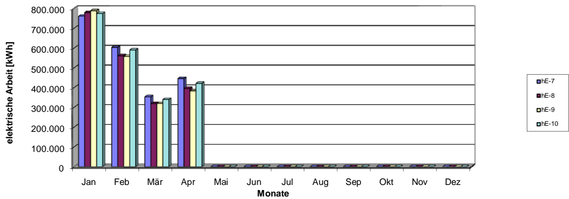
Ertrag 2012 - hessenWIND VI - Helpershain-Meiches
